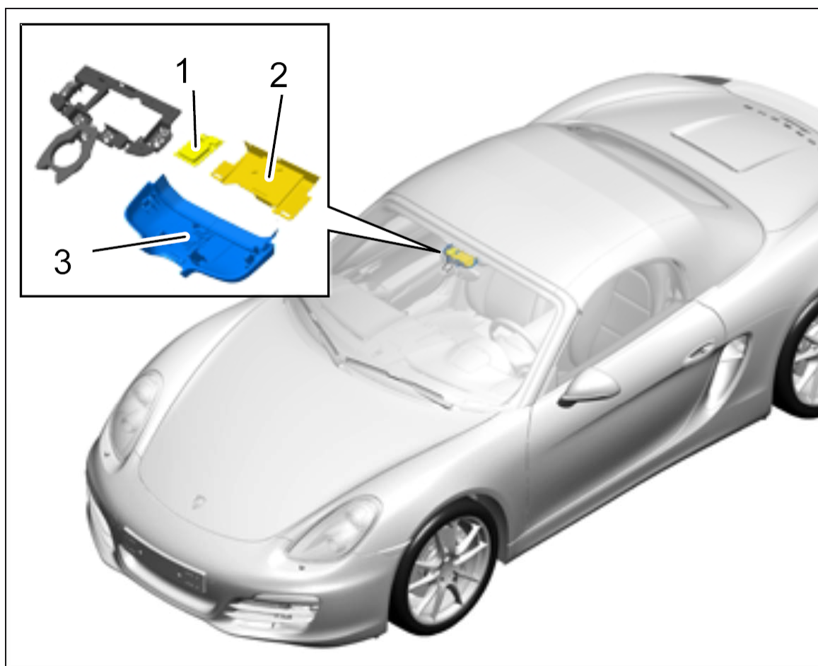
GPS 天线的安装位置
