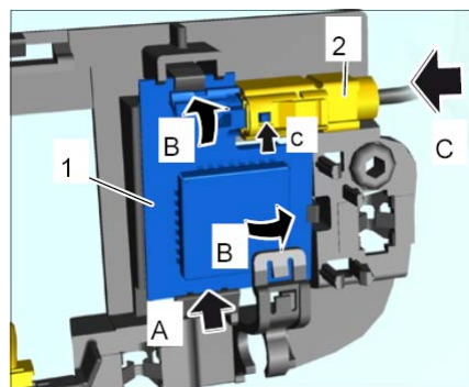
安装 GPS 天线
