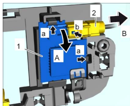
拆卸 GPS 天线
