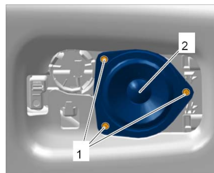
拆卸后部音箱
