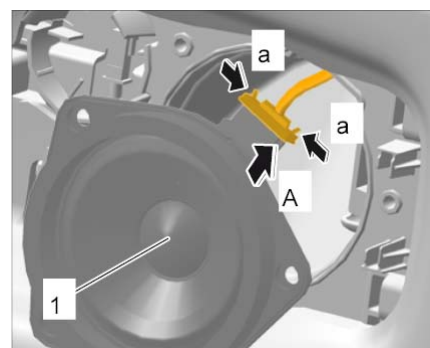
断开后部音箱的电气插头
