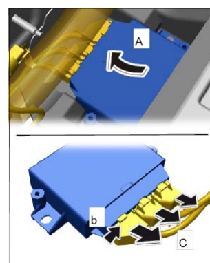
拆卸控制单元
