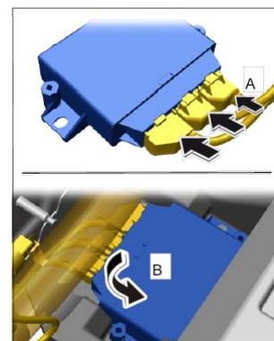
安装控制单元
