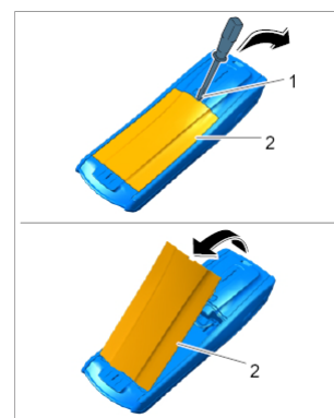
打开盖子
