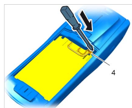
安装蓄电池
