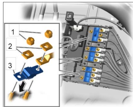
固定乘客舱内的保险熔丝
