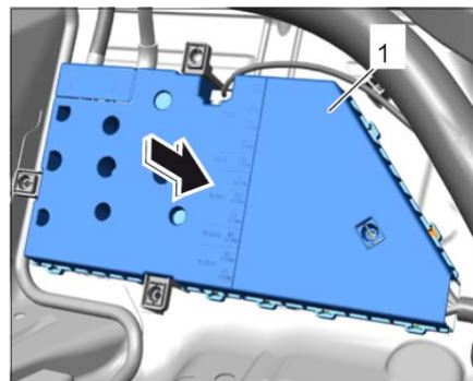
固定乘客舱中的电源分配器盖
