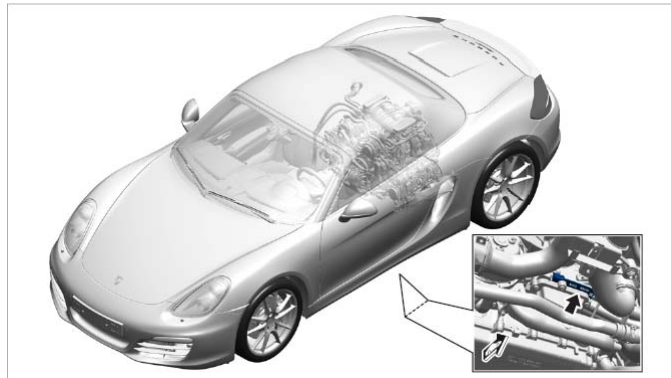
发动机号在车辆上的位置
