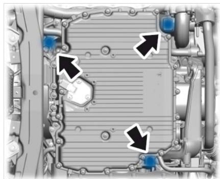
发动机支承点
