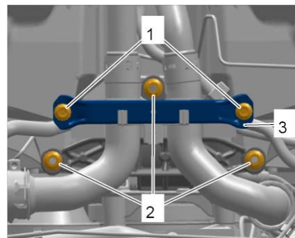
发动机支承和冷却液软管保持架
