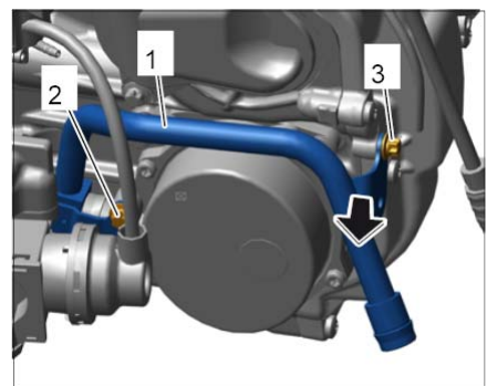
松开刚性真空管路
