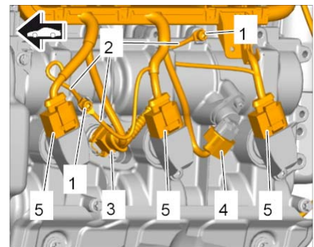
气缸盖上的接地线和插头
