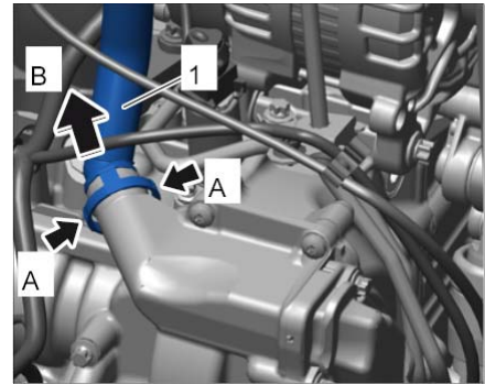
松开曲轴箱强制通风软管
