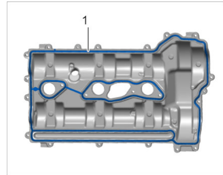
气缸盖罩 4-6 上的密封件
