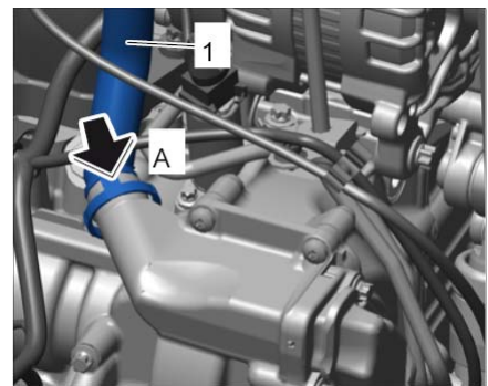
推上曲轴箱强制通风软管，直到其接合。
