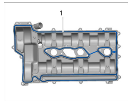
气缸盖罩 1-3 上的密封件
