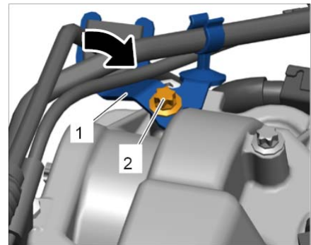
固定燃油管路的保持架
