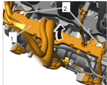
松开喷油器的电缆扎带
