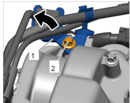
松开燃油管路的保持架
