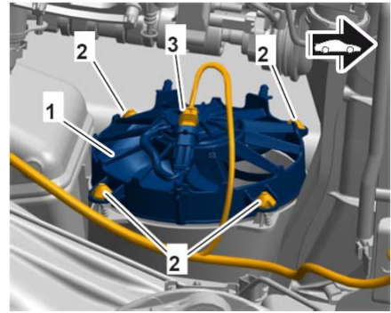
从下面安装发动机舱风机
