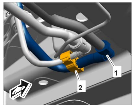
管路托架
