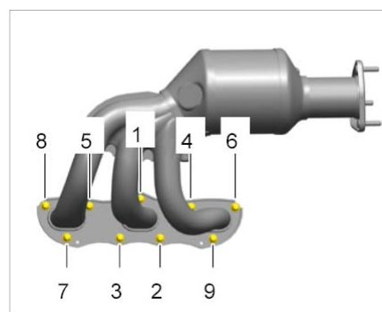
排气歧管的紧固顺序
