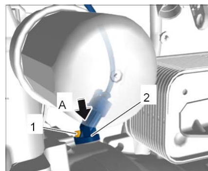
安装曲轴脉冲传感器
