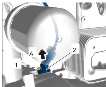
拆下曲轴脉冲传感器
