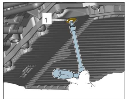
放油塞
