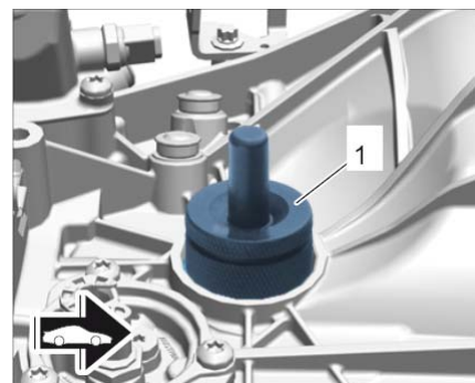
安装密封环
