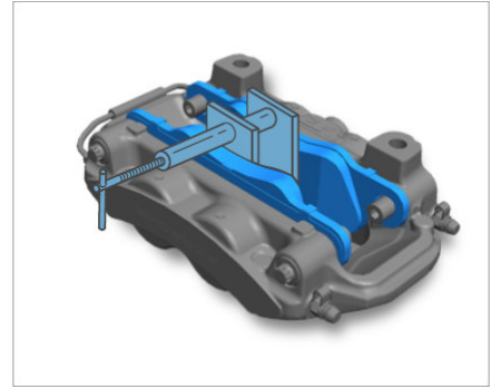
压回制动片
