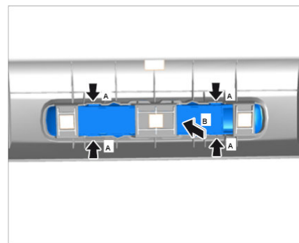
拆卸释放装置
