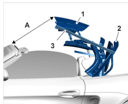
处于维修位置的软篷
