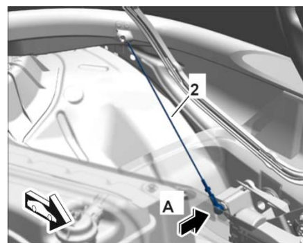
接合张紧绳
