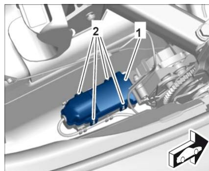
拆卸上饰板
