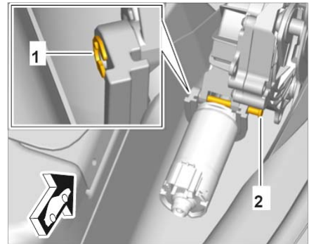
安装固定销
