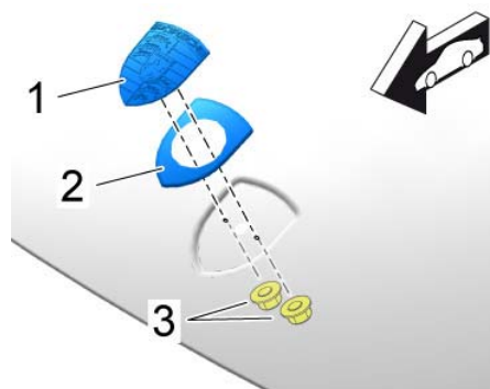
拆下徽标和底座
