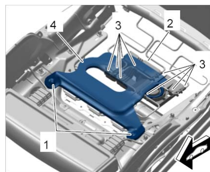
安装压力传感器垫
