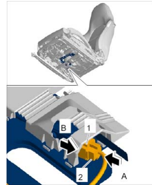
插入并锁定电气插头
