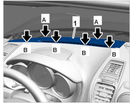
安装仪表板盖（除霜器饰件）
