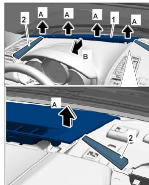
拆卸仪表板盖（除霜器饰件）
