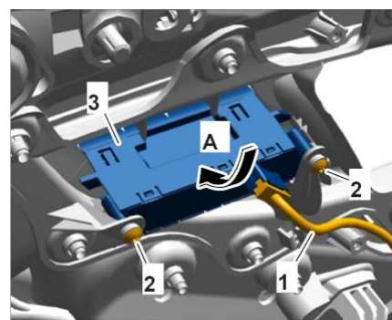
固定记忆座椅调节开关
