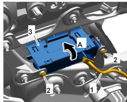
断开记忆座椅调节开关
