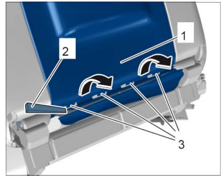
松开后罩
