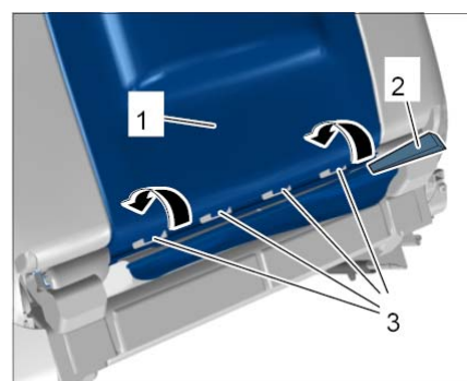
固定座椅罩
