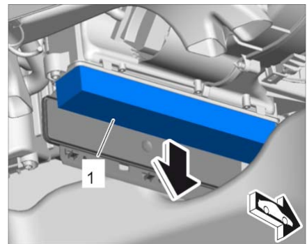
拔出微粒过滤器
