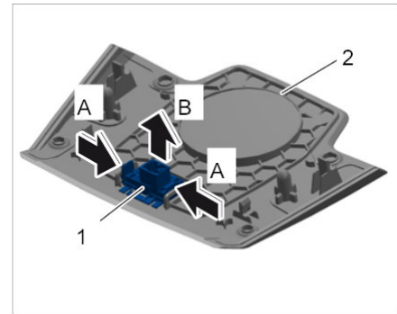
拆卸日照传感器
