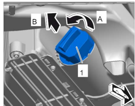
拆卸风扇控制按钮
