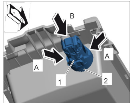
拆卸插座
