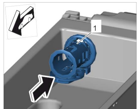
安装插座
