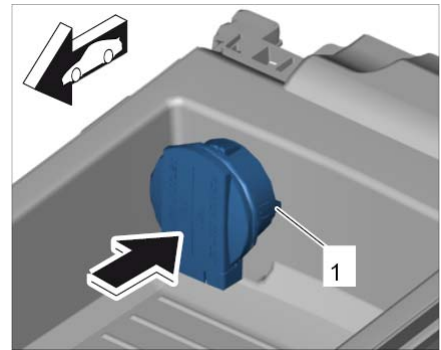
安装带罩的紧固环
