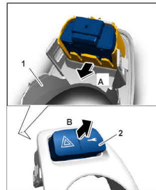
拆卸警示灯开关
