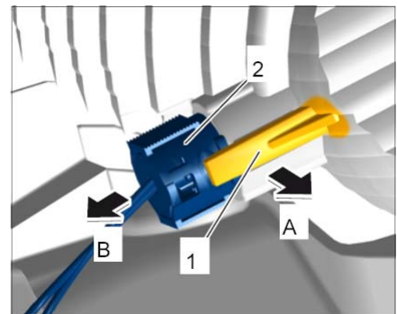
拆卸壳体
