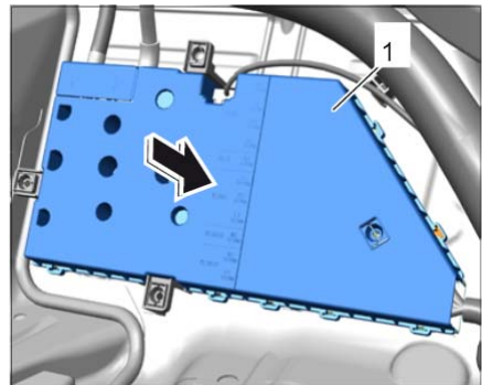
固定乘客舱中的电源分配器盖
