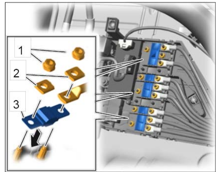
固定乘客舱内的保险熔丝
