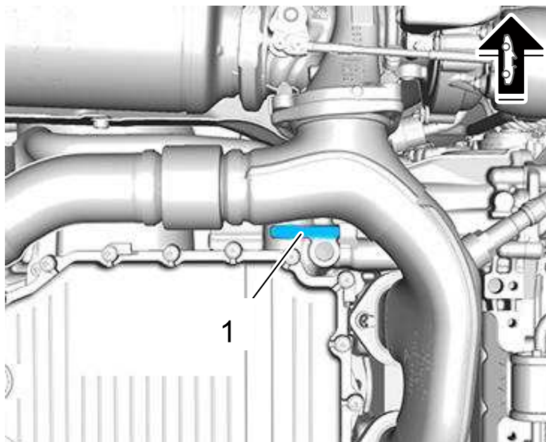
发动机号的位置
