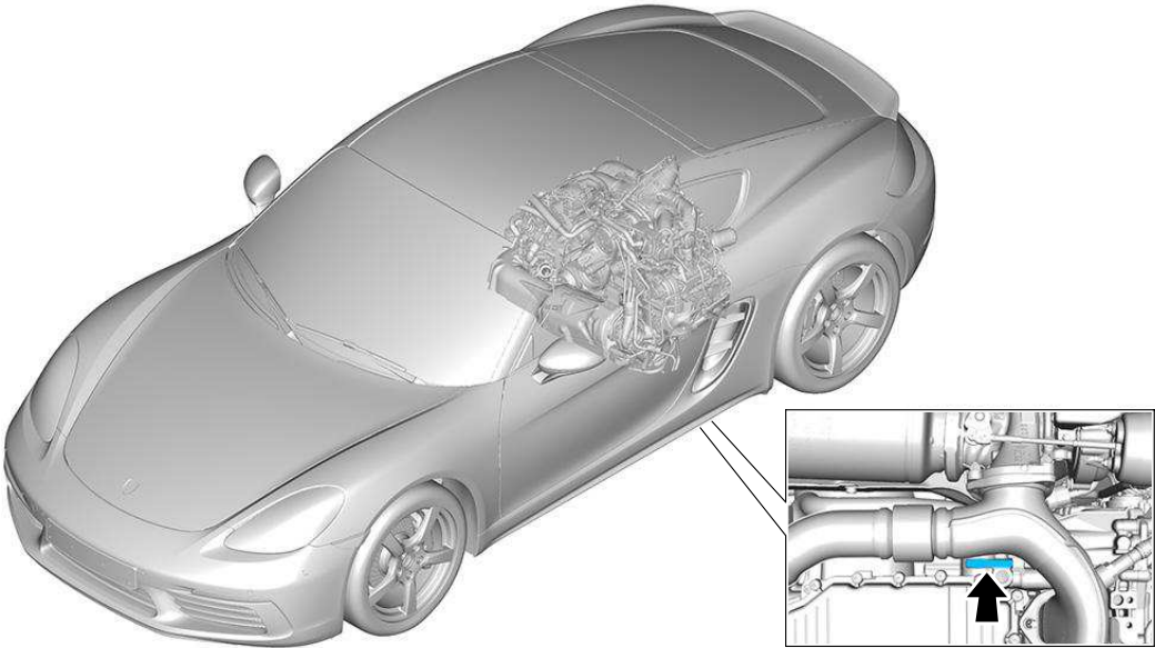
发动机号在车辆上的位置
