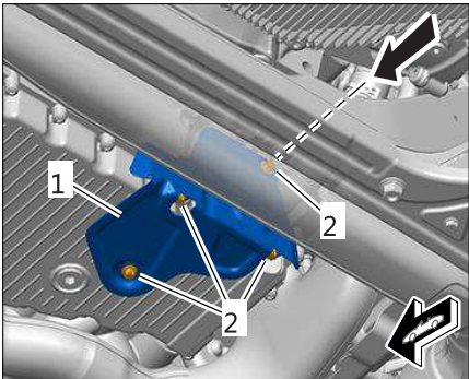
油底壳下部的隔热板
