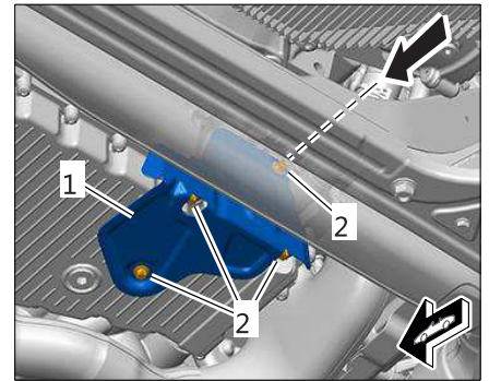
油底壳下部的隔热板
