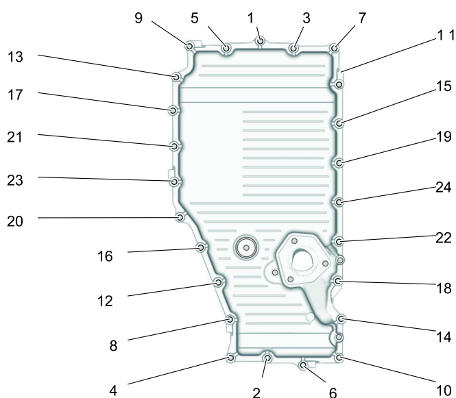
将油底壳下部固定到油底壳上部的紧固顺序
