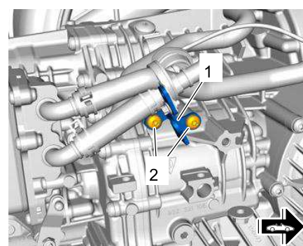
冷却液调节器支架
