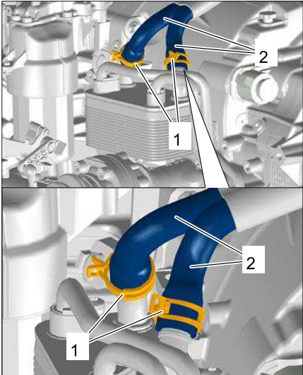
断开冷却液软管
