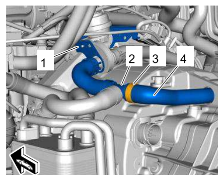
PDK 附加零件
