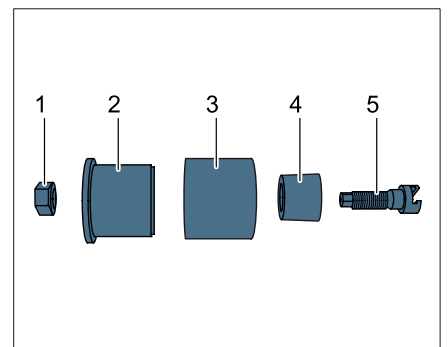
Porsche Doppelkupplung (PDK) 保时捷双离合器变速箱径向轴密封件的装配工具
