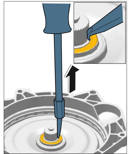
拆卸密封环
