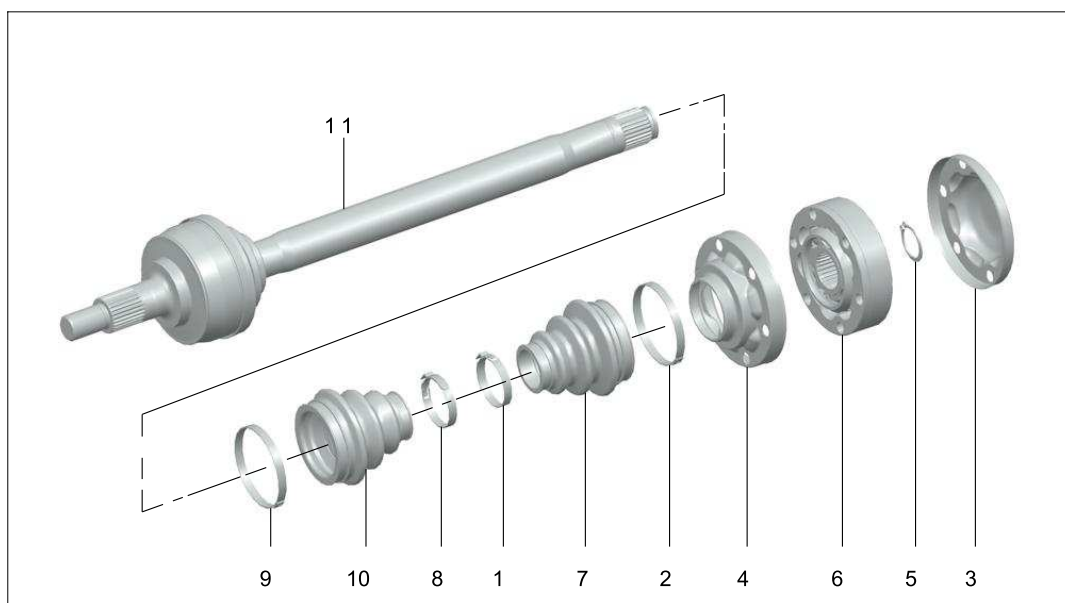
驱动轴已拆解
