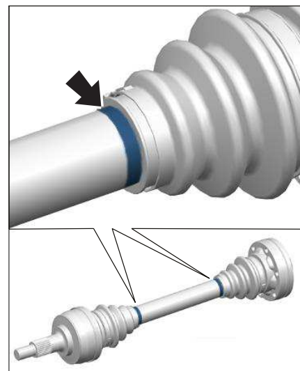
标记驱动轴上防尘套的位置
