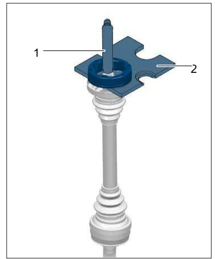
压出等速万向节
