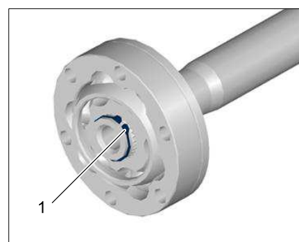
拆卸挡圈
