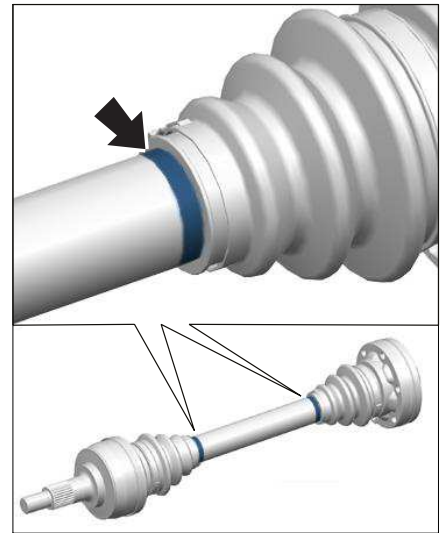
标记驱动轴上防尘套的位置
