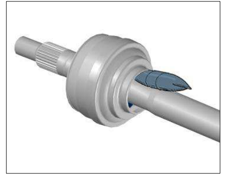
为车轮侧的等速万向节涂抹润滑脂
