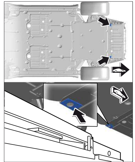
前桥高度测量点
