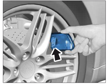
检查制动片
