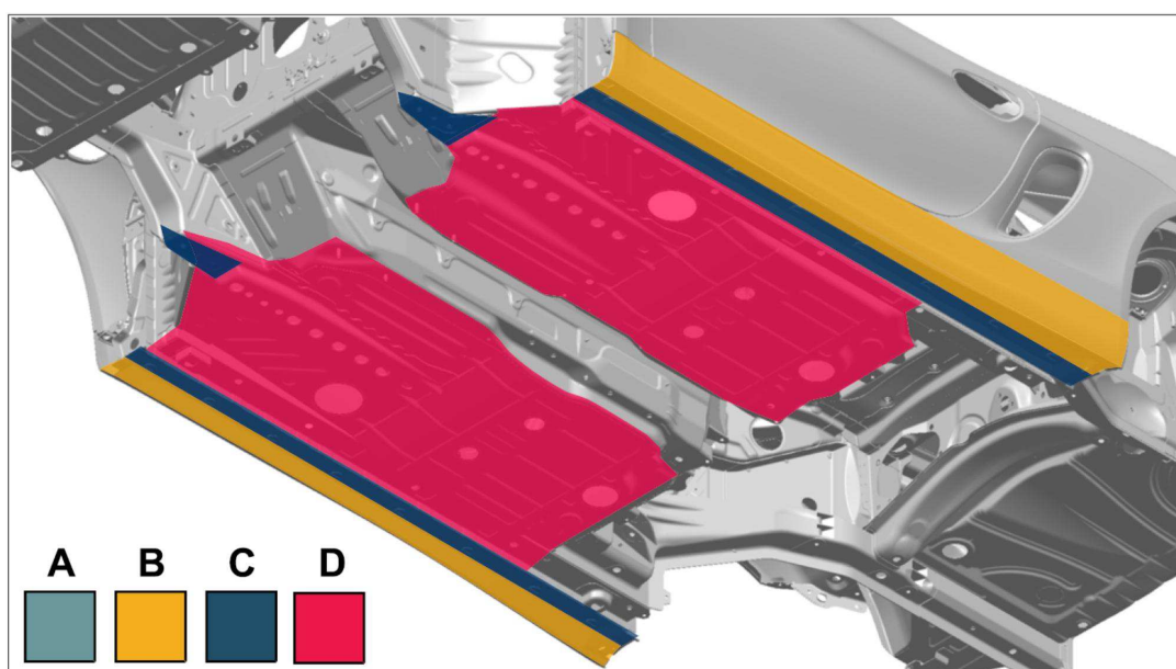
概图 - 下侧梁和地板
