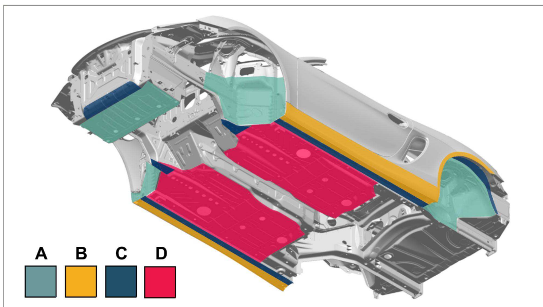
概图 - 车底防护
