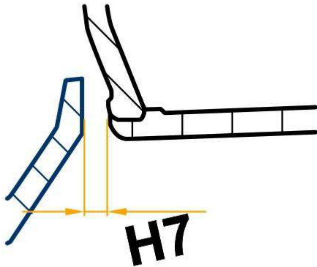
主大灯的间隙尺寸
