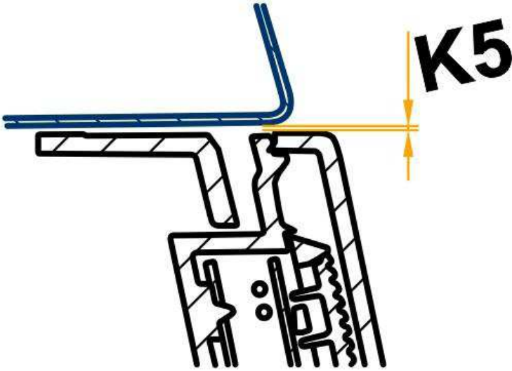
前翼子板的间隙尺寸
