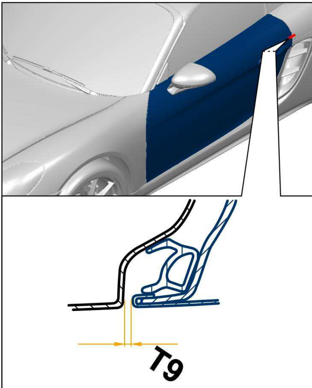
前车门的间隙尺寸
