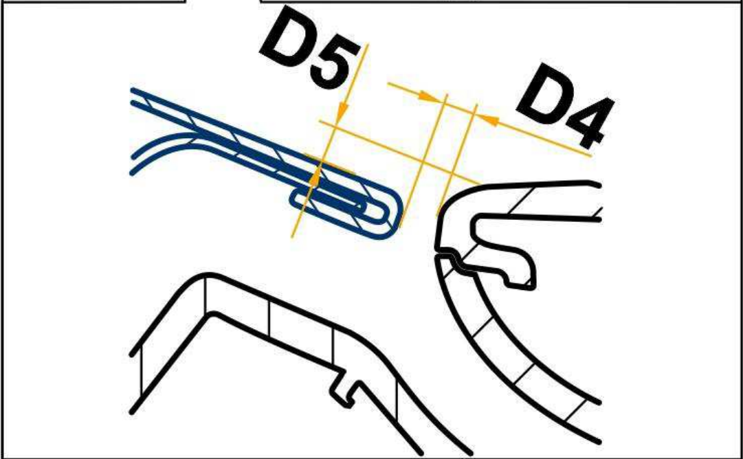
后盖的间隙尺寸
