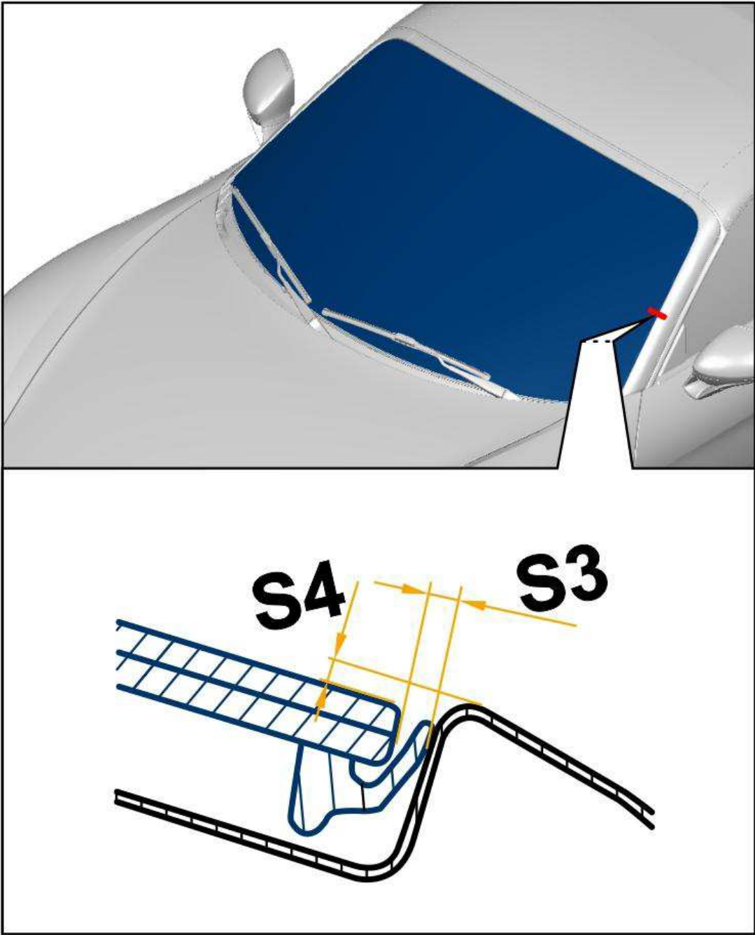
挡风玻璃的间隙尺寸
