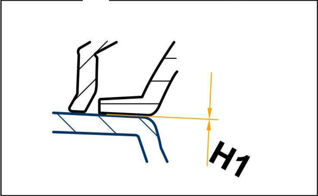
后裙板的间隙尺寸
