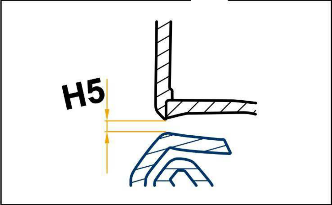
主大灯的间隙尺寸
