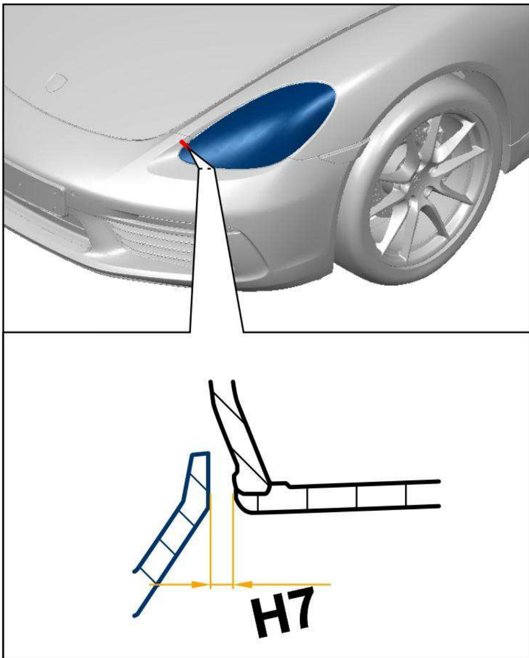
主大灯的间隙尺寸
