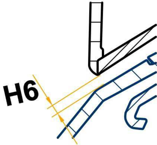
主大灯的间隙尺寸
