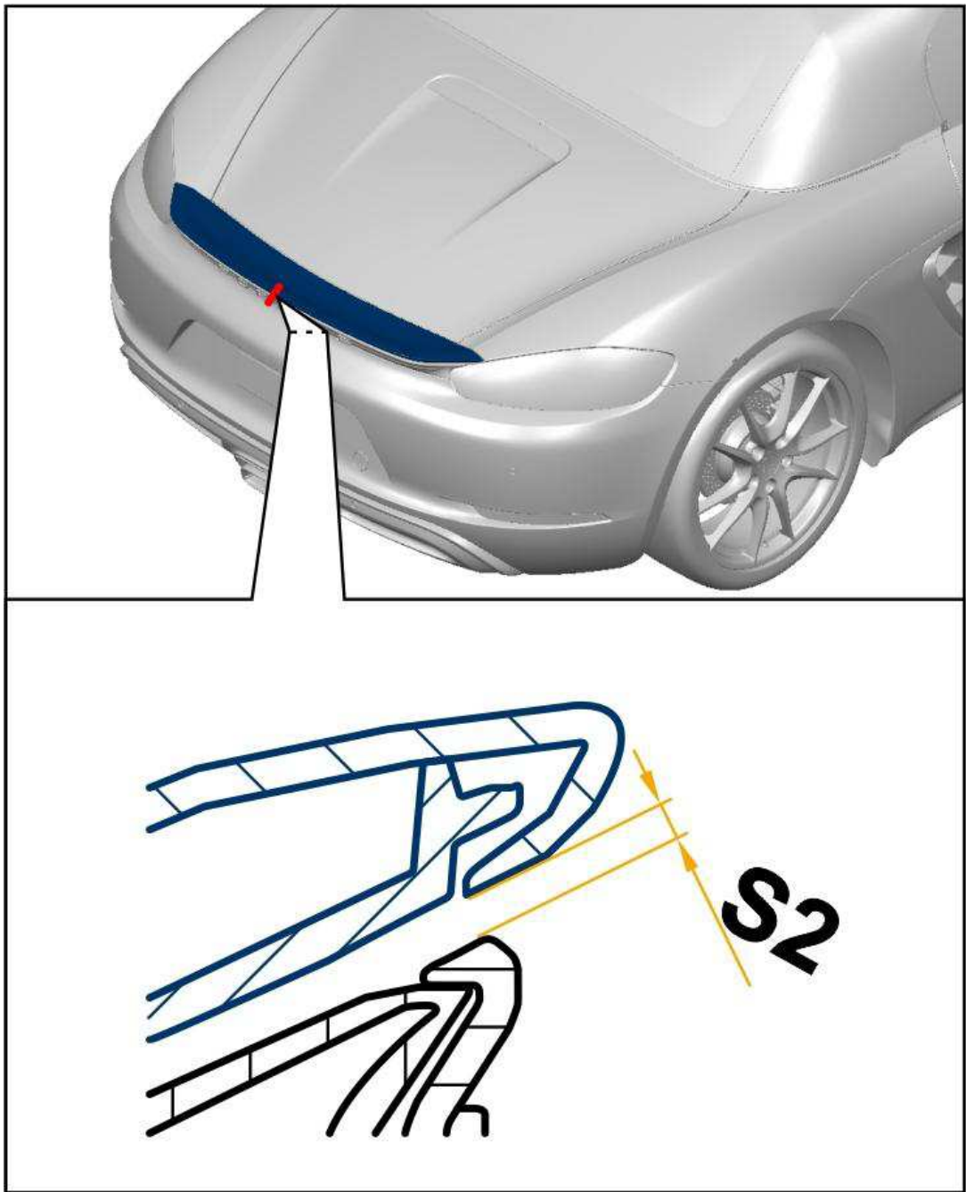
后扰流板的间隙尺寸
