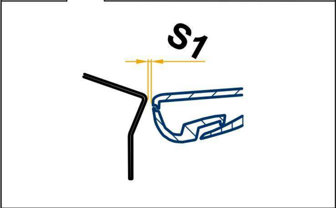
后扰流板的间隙尺寸
