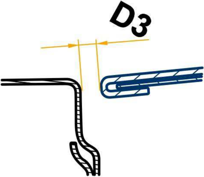
后盖的间隙尺寸
