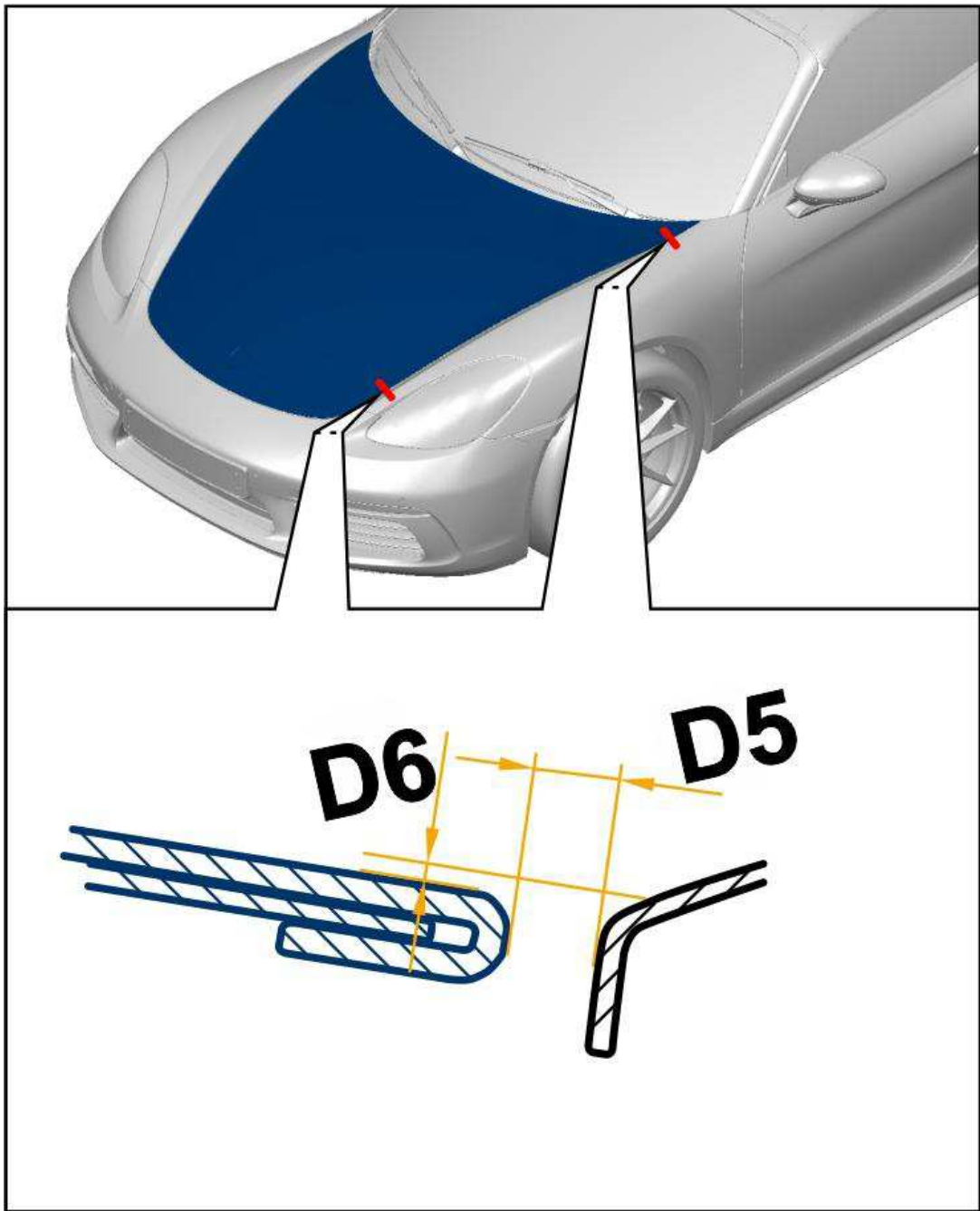
前盖的间隙尺寸
