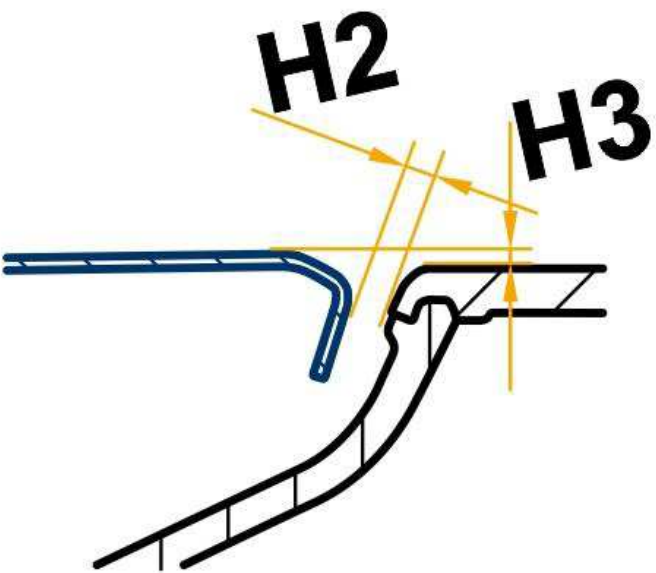
主大灯的间隙尺寸
