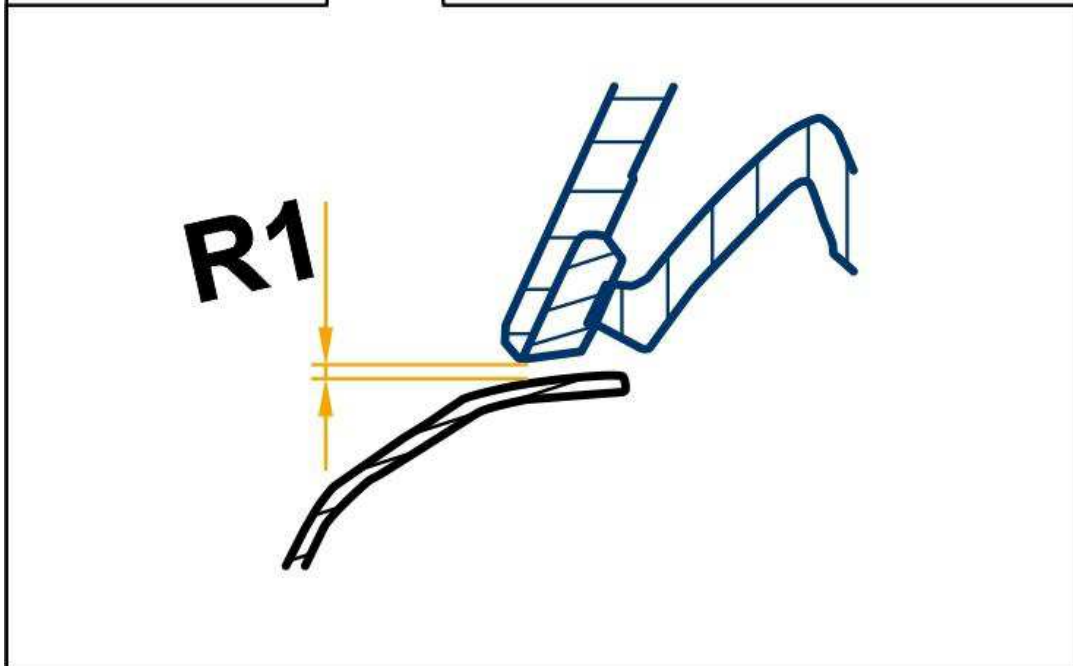
尾灯间隙尺寸
