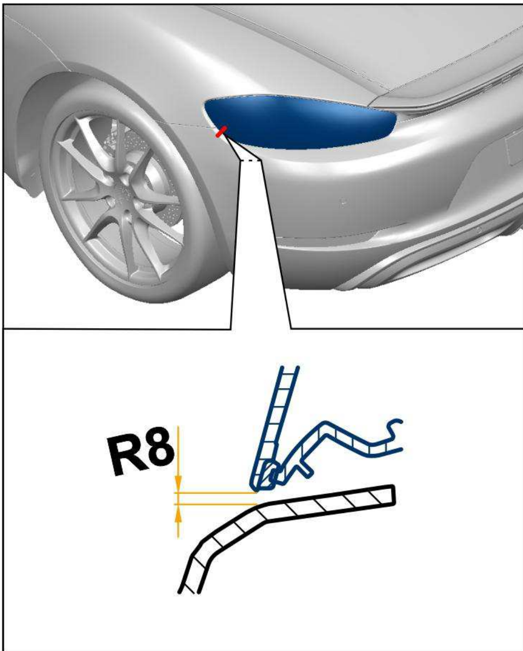
尾灯间隙尺寸
