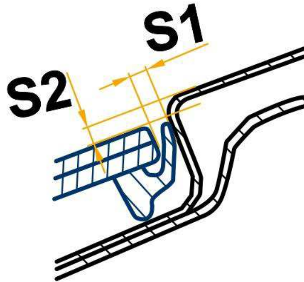
挡风玻璃的间隙尺寸
