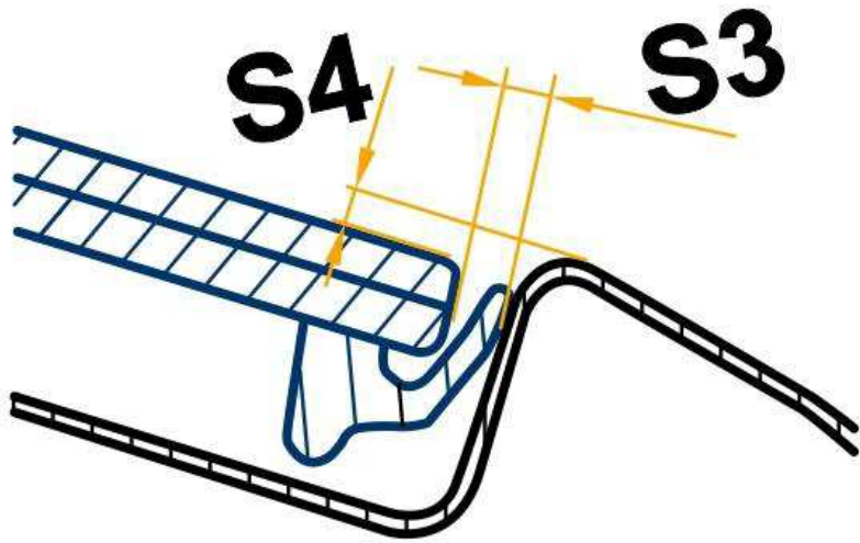
挡风玻璃的间隙尺寸
