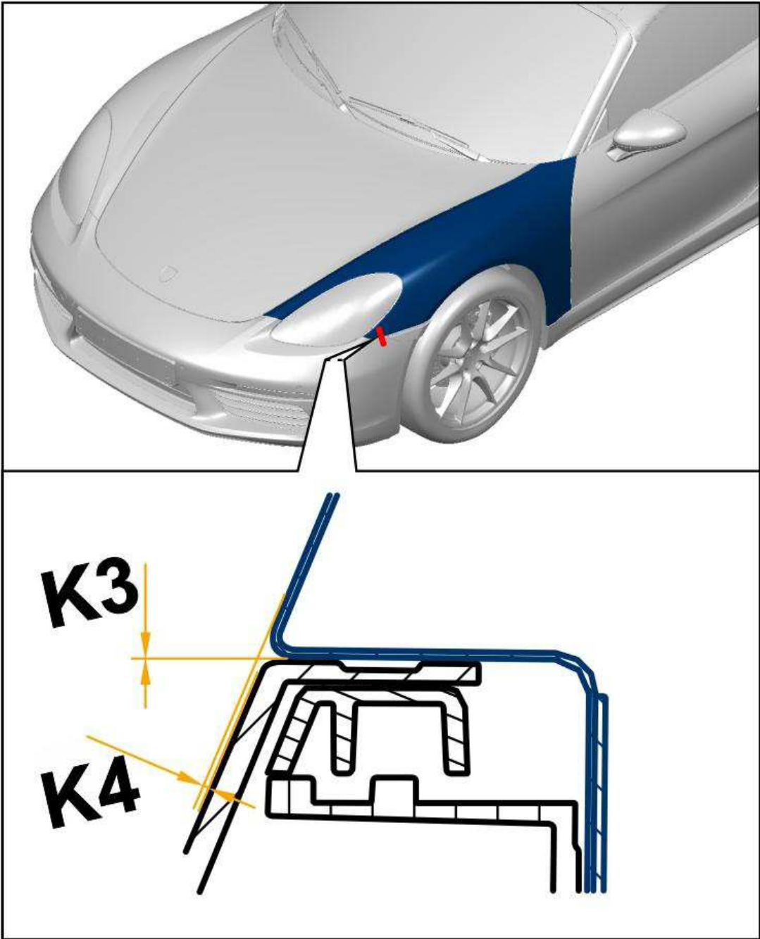
前翼子板的间隙尺寸
