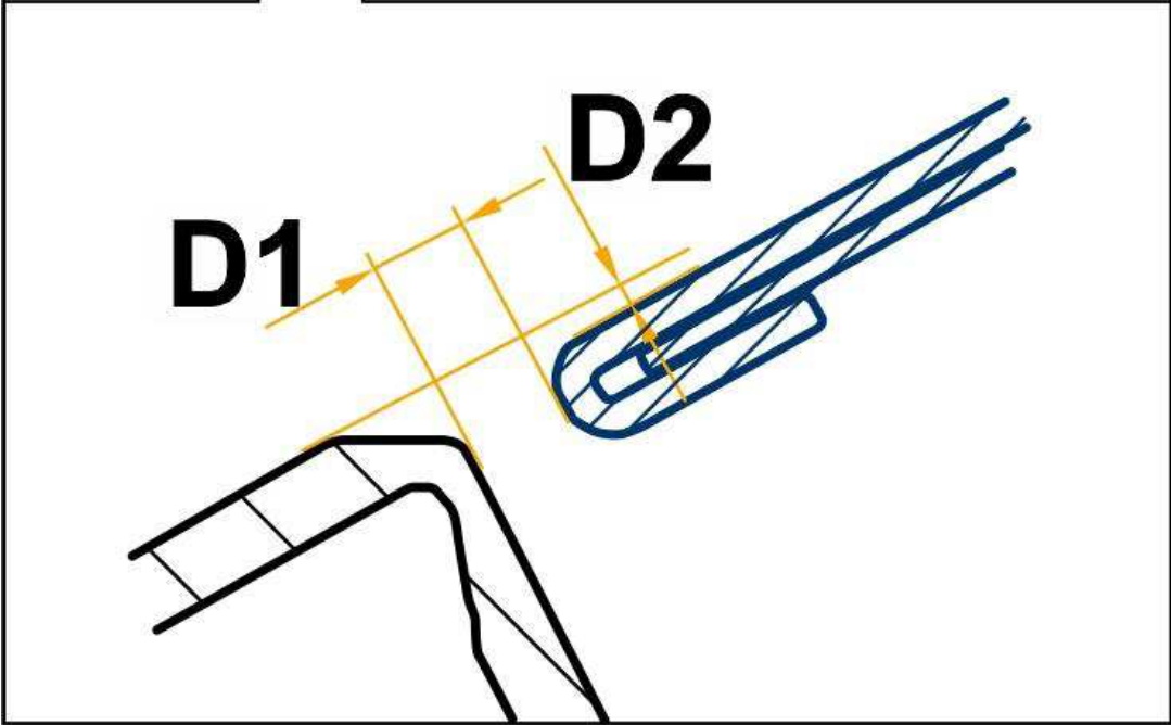
前盖的间隙尺寸
