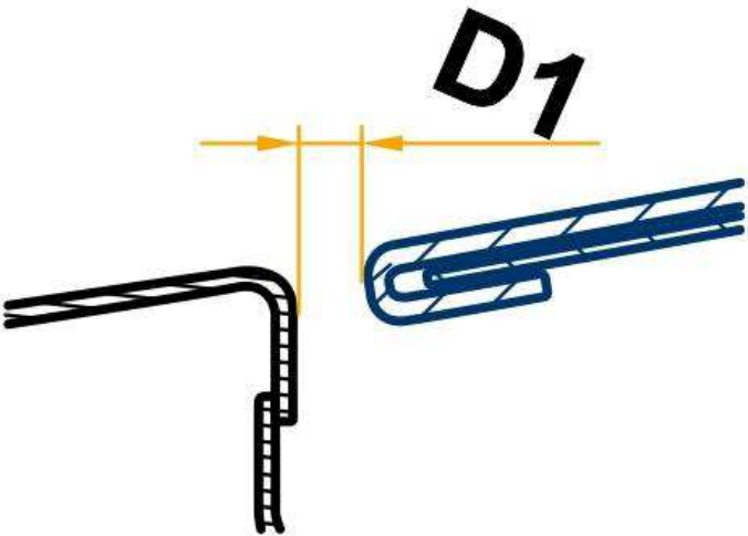
后盖的间隙尺寸
