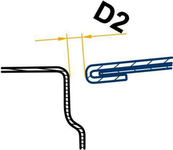
后盖的间隙尺寸
