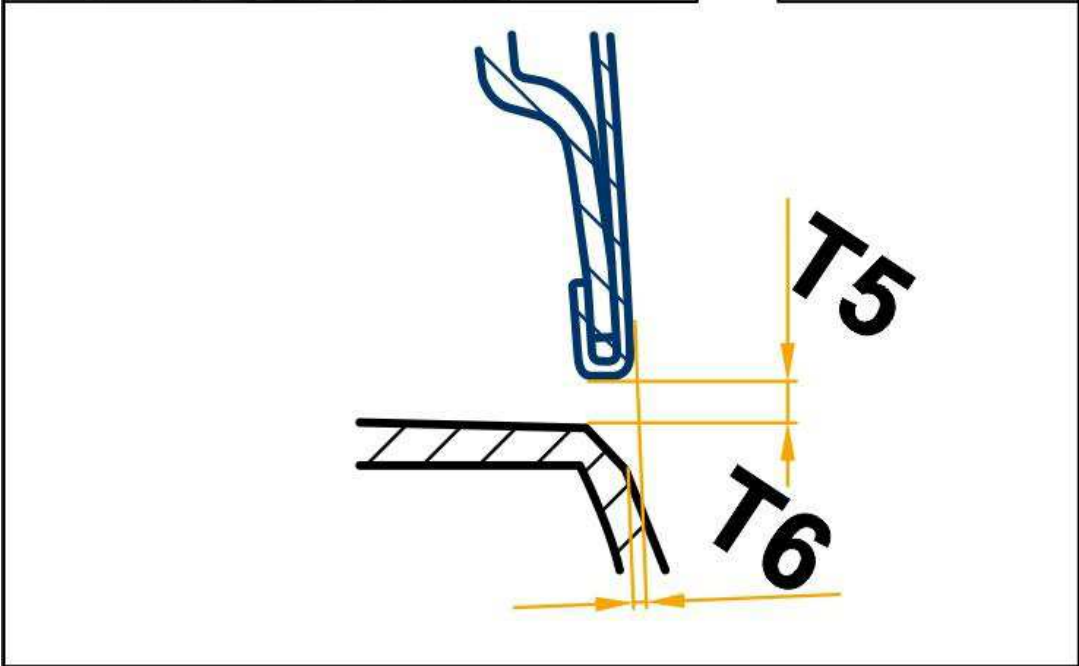
前车门的间隙尺寸
