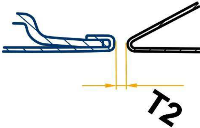
前车门的间隙尺寸
