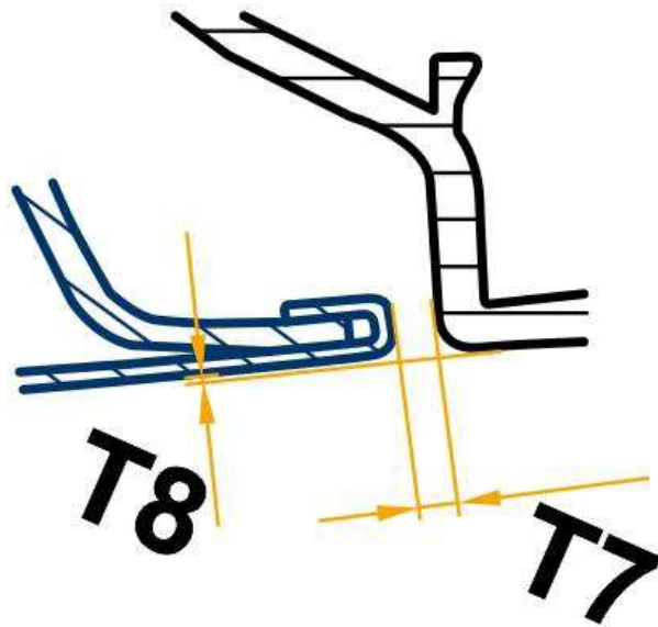
前车门的间隙尺寸
