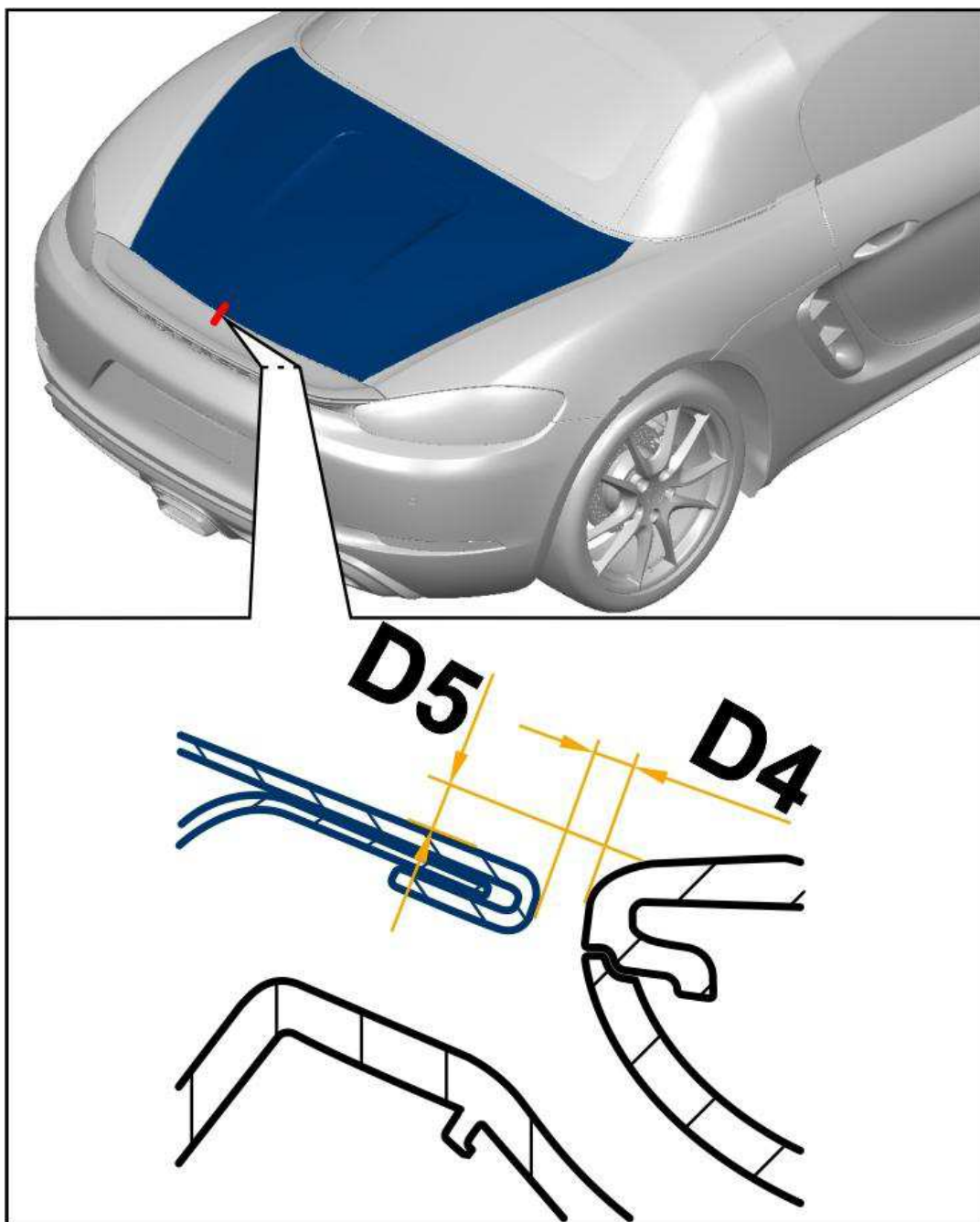
后盖的间隙尺寸
