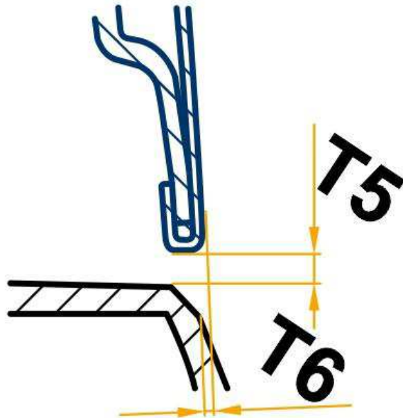
前车门的间隙尺寸
