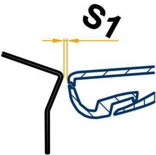
后扰流板的间隙尺寸
