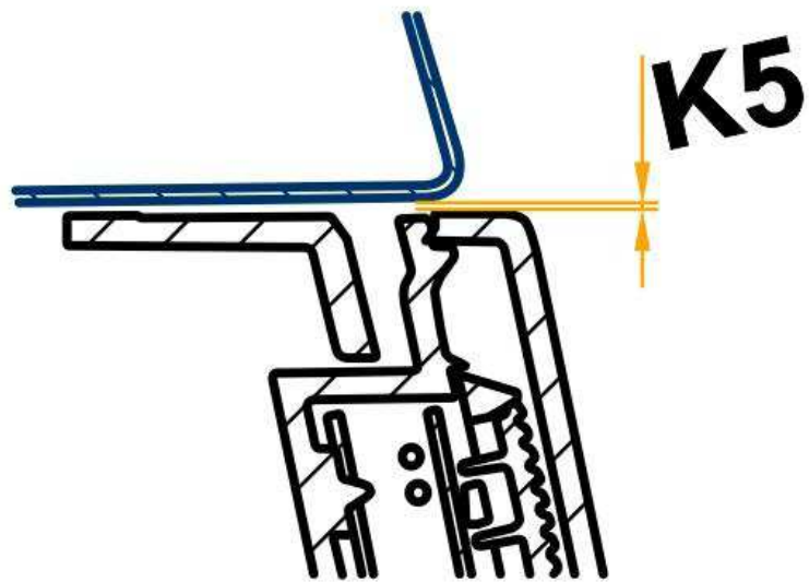
前翼子板的间隙尺寸
