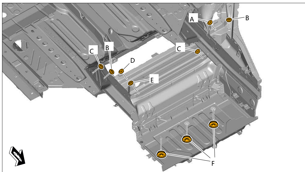
下部车身前部
