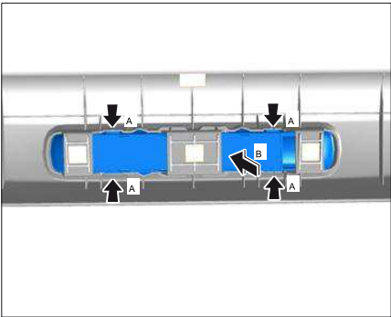
拆卸前盖解锁装置
