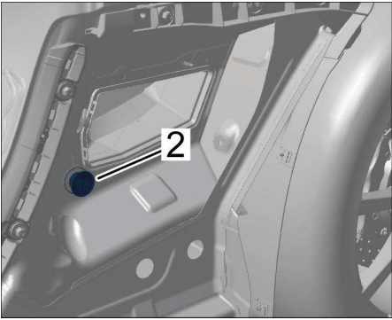
拆卸排水软管阀
