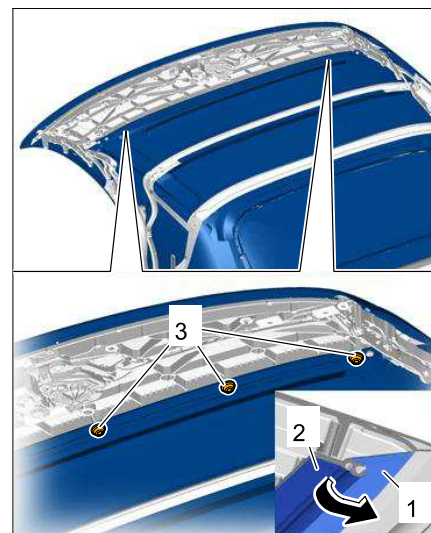
松开束带
