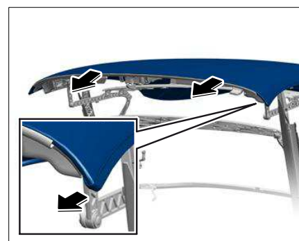
拆卸活动顶篷罩
