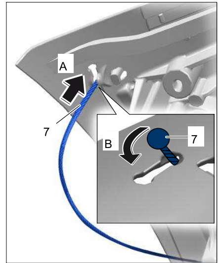
分离张紧绳
