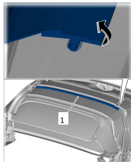
拆下前车顶支柱处的活动顶篷盖罩
