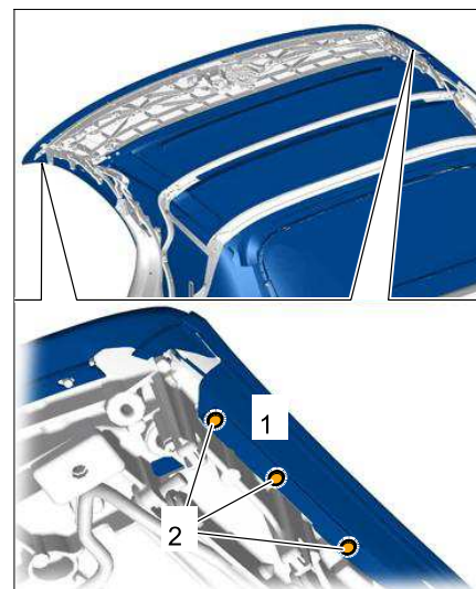
前外侧铆钉
