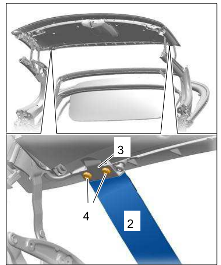
松开拉力带
