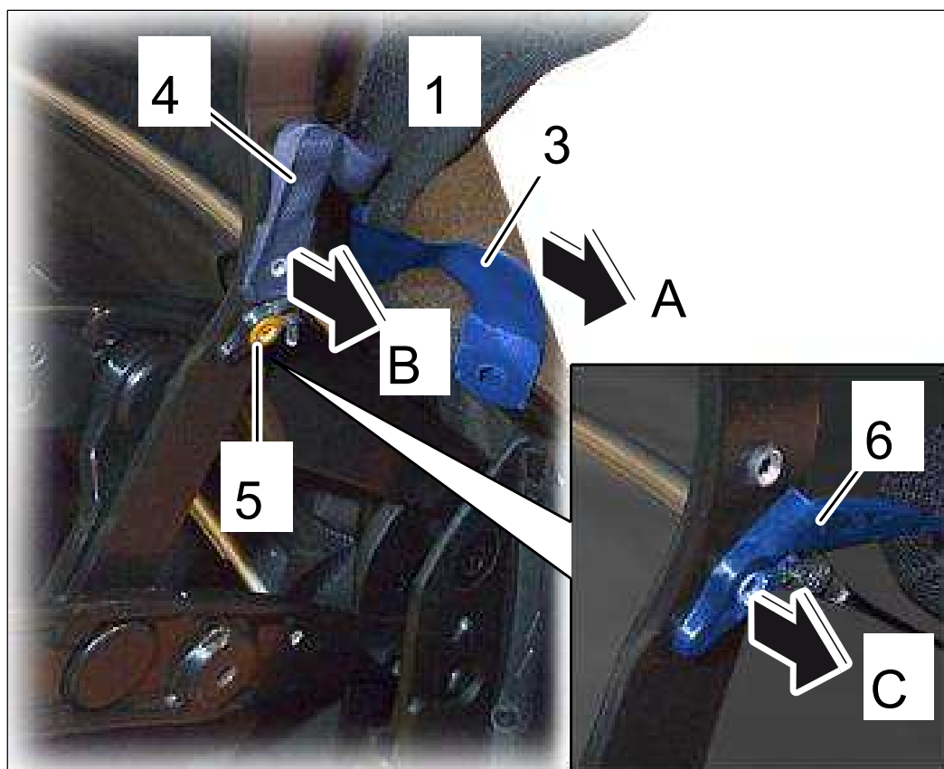
拆下折叠放置装置绳索
