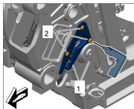
拆卸微动开关
