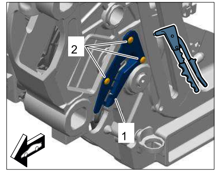
安装微动开关
