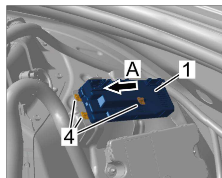
拆卸活顶控制单元
