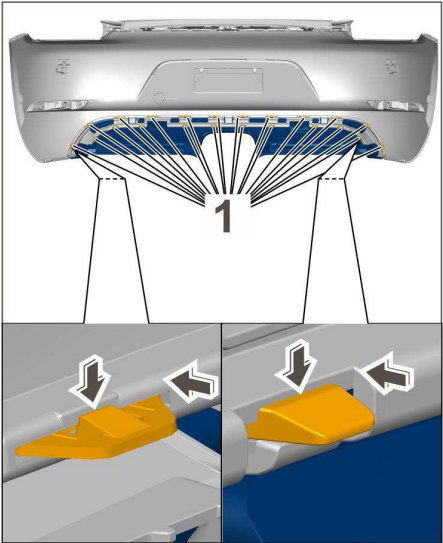
固定卡子
