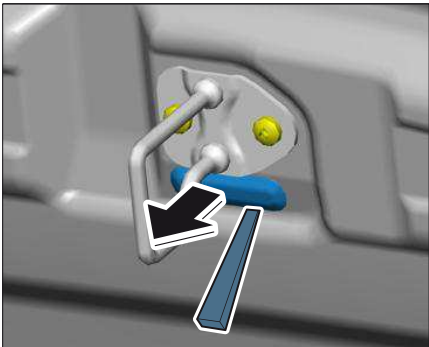
松开护盖
