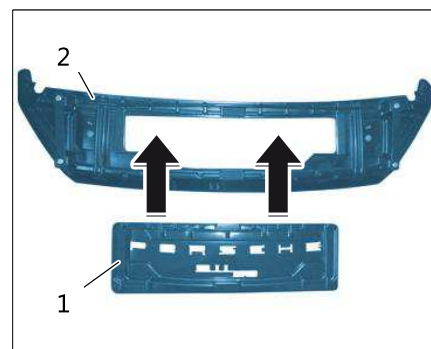
准备标志模板 (以 991 为例)
