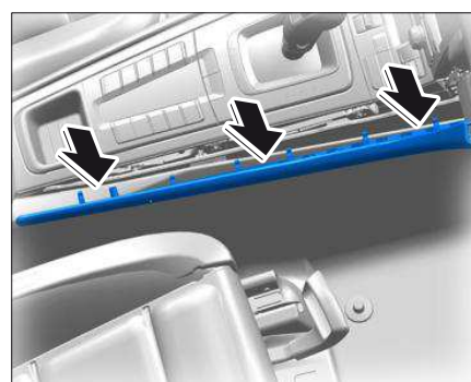
松开侧饰板
