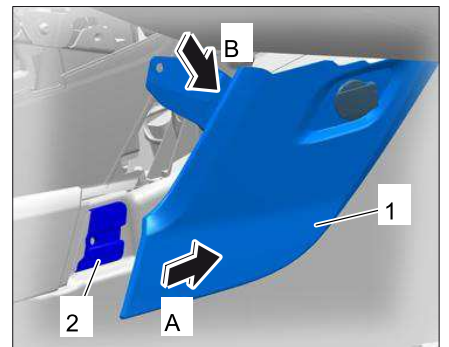
拆卸脚坑出风口饰件
